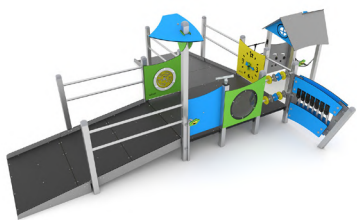
PERCORSO WASHINGTON VIN1726 642x525 cm h. 231 cm 942x825 cm TÜV EN 1176:2017
