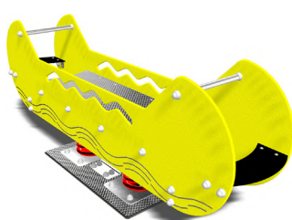
MOLLONE CANOA SYNRA 210x40 cm h. 80 cm 410x240 cm EN 1176:2017
