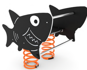
MOLLONE SQUALO BIPOSTO VIN0623 79x78 cm h. 78 cm 374x322 cm TÜV EN 1176:2017
