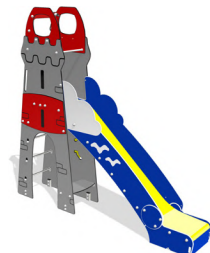
SCIVOLO TORRE MEDIOEVALE SYNTPH 300x60 cm h. 280 cm 542x352 cm EN 1176:2017
